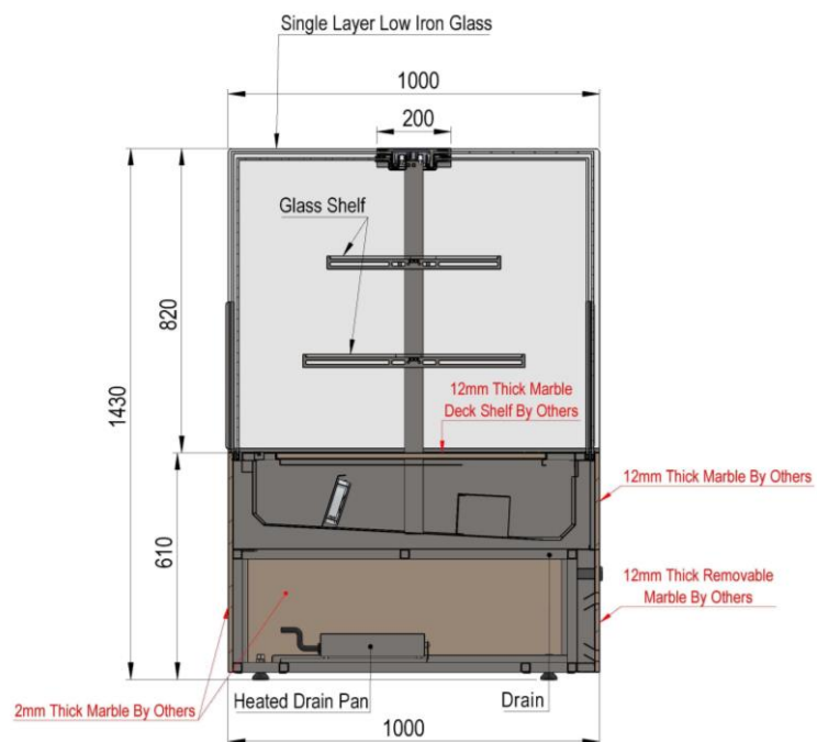
SECTION D-D SCALE 1 : 13
